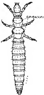
Fig. 110. Eosentomen ribagai Berlese.
